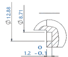
局部视图 C 比例 2:1
